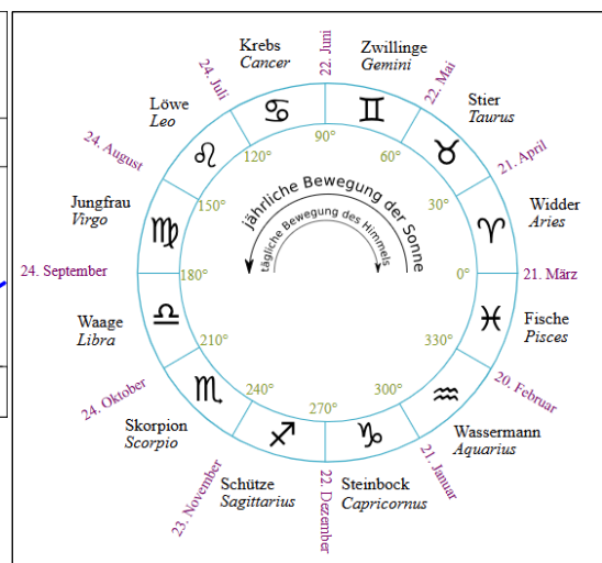
Abb. 2 Links: Schematische Darstellung der Sternbilder und Tierkreiszeichen. Rechts: Kreisförmige Darstellung des Tierkreises mit den 12 einzelnen Tierkreiszeichen. In der Bildmitte sind die jährliche Bewegung der Sonne und die tägliche Bewegung des Himmels dargestellt. (Alsterblick, Bild-frei/Gemeinfrei; WolfgangRieger, Gemeinfrei; je Wikimedia)
