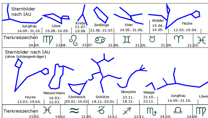
Abb. 2 Links: Schematische Darstellung der Sternbilder und Tierkreiszeichen. Rechts: Kreisförmige Darstellung des Tierkreises mit den 12 einzelnen Tierkreiszeichen. In der Bildmitte sind die jährliche Bewegung der Sonne und die tägliche Bewegung des Himmels dargestellt. (Alsterblick, Bild-frei/Gemeinfrei; WolfgangRieger, Gemeinfrei; je Wikimedia)
