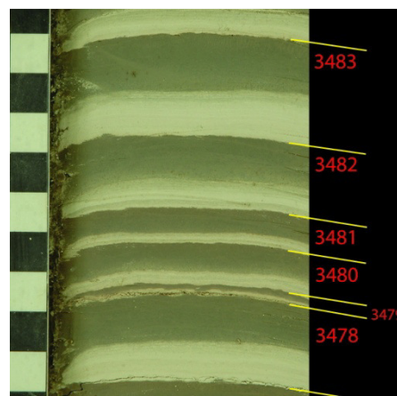
Abb. 1 Bänderton, Connecticut Valley, USA.
